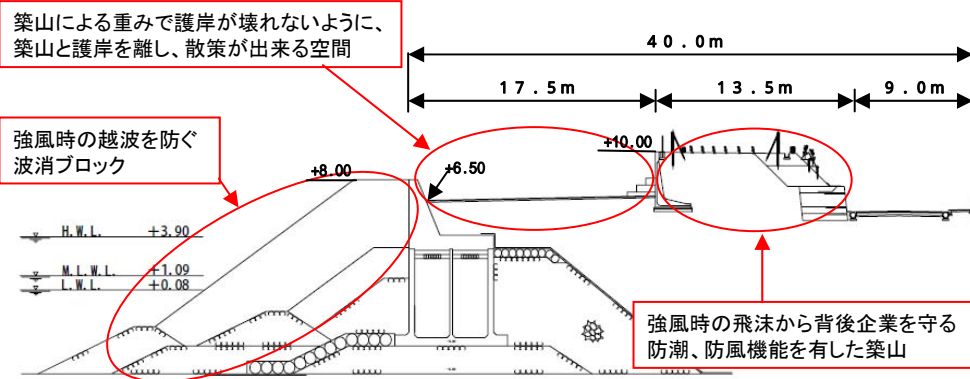
標準断面図
